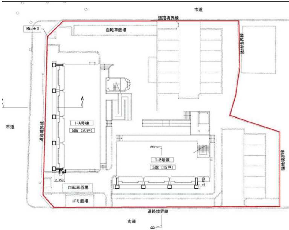
1号棟 配置図
